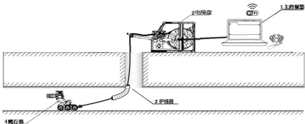
图 3-1 检测流程图
