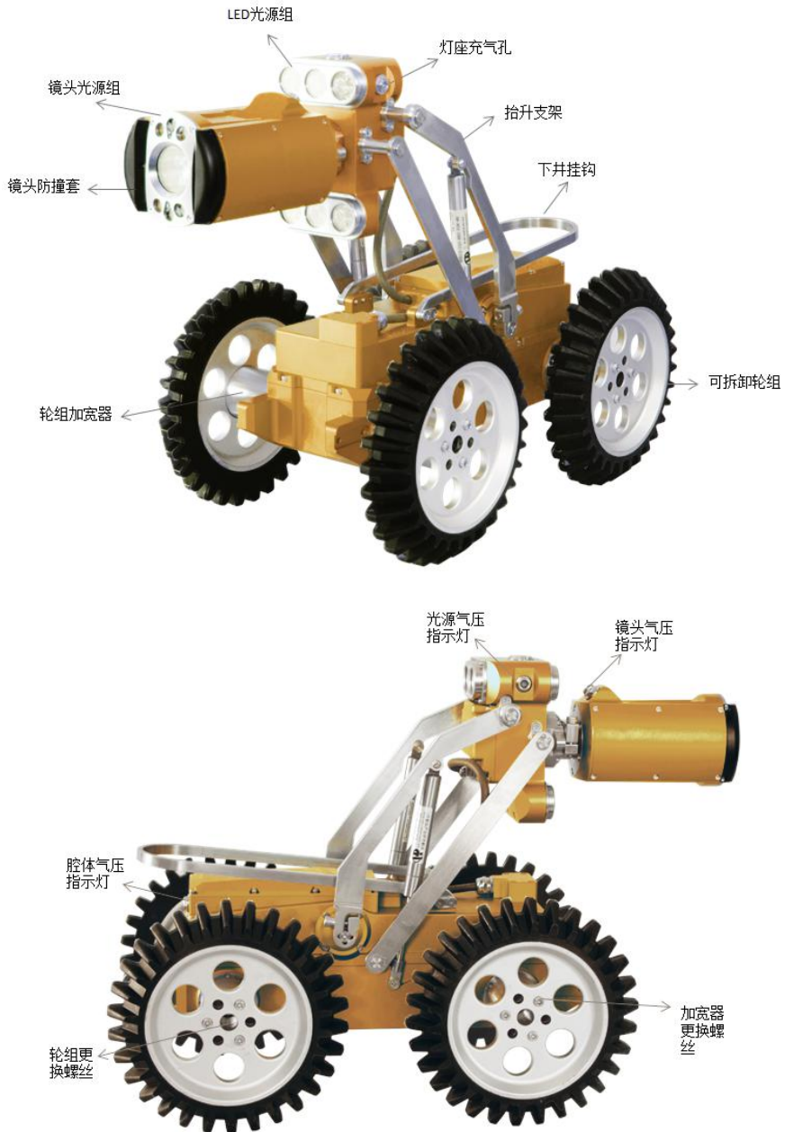
图 2-2 爬行器
