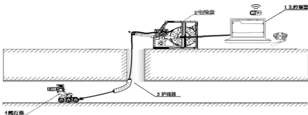
图 2-1 现场施工图
